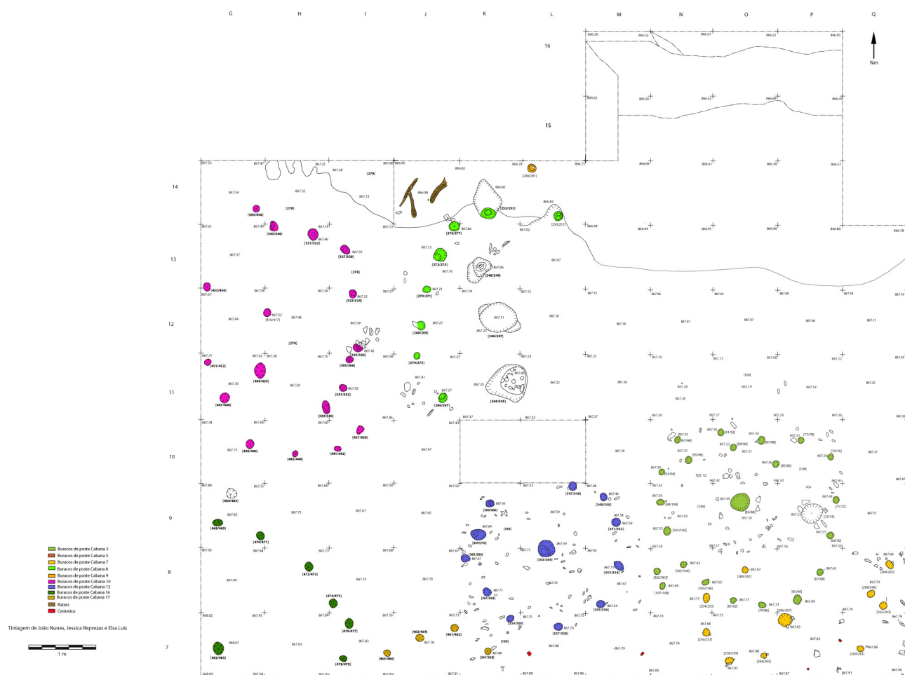
Fig. 3 – Planta ao nível da interface superior da UE. 109=278, com as estruturas negativas das Fases 1 e 2 detectadas. “Cabanais”, 3, 7, 8, 10, 12, 16 e 17.
