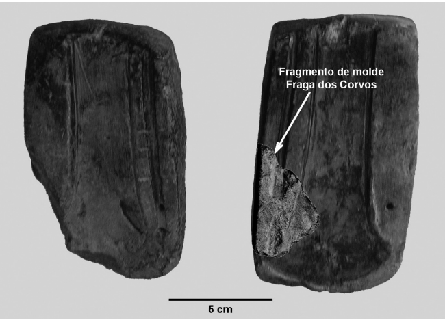
Fig. 11 – Fraga dos Corvos, Macedo de Cavaleiros. Fragmento de Molde para machados Bujões/Barcelos e cinzeis [FCORV-A 2220] sobreposto ao molde completo do Museu de Orense.
