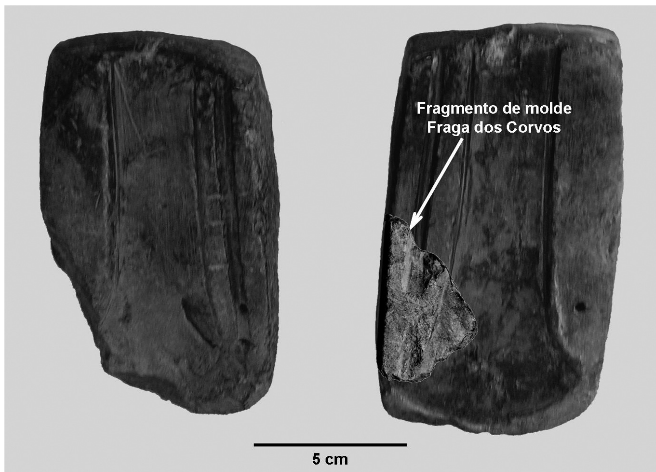
Fig. 8 – Fraga dos Corvos, Macedo de Cavaleiros. Fragmento de Molde para machados Bujões/Barcelos e cinzeis [FCORV-A 2220] sobreposto ao molde completo do Museu de Orense.
